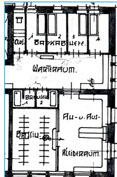
Abb. 3: Das ursprüngliche Raumlayout des Volksbades im neuen Schulhaus.
